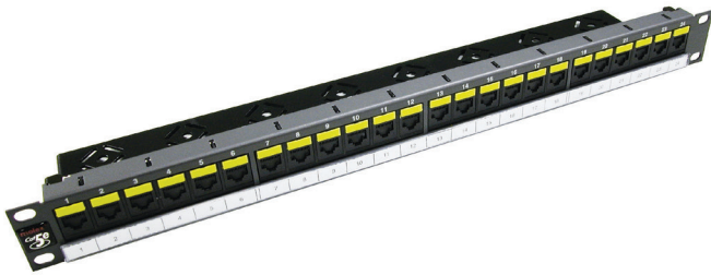
1U 24口 PowerCat 5e 配线架 尺寸: 44mm x 483mm x 98mm 包装重量: 978.6g
