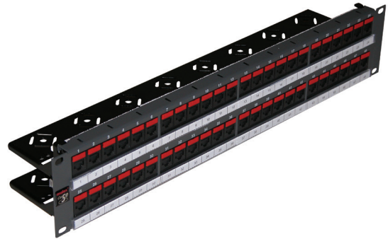
2U 48口 PowerCat 5e 配线架 尺寸: 88mm x 483mm x 98mm 包装重量: 1504.5g
